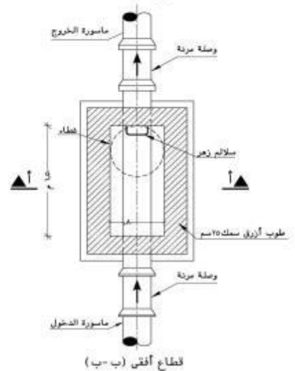
شكل رقم (٢-١٥): تفاصيل مطابق الشوارع الضيقة.
