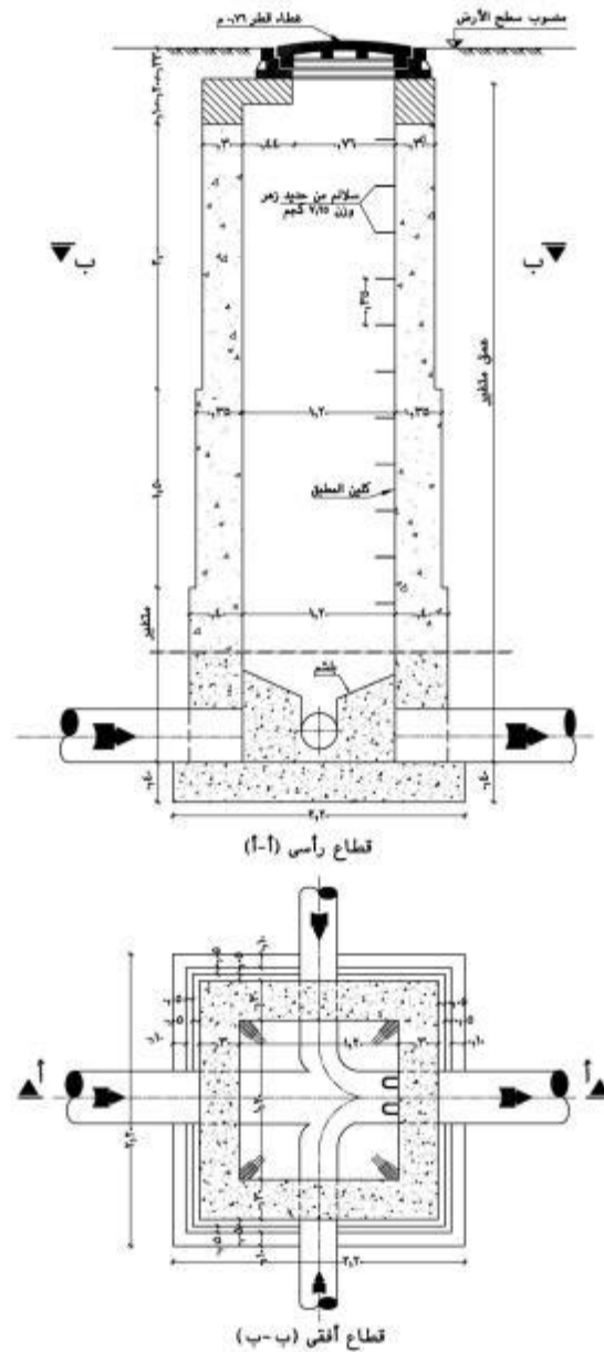
شكل رقم (٢-٨): تفاصيل المطبق المربع من الخرسانة العادية لعق أكبر من ٤,٥٠ متر ولمواسير بقطر أكبر من ٤٠٠ وأقل من ٩٠٠ مم.
