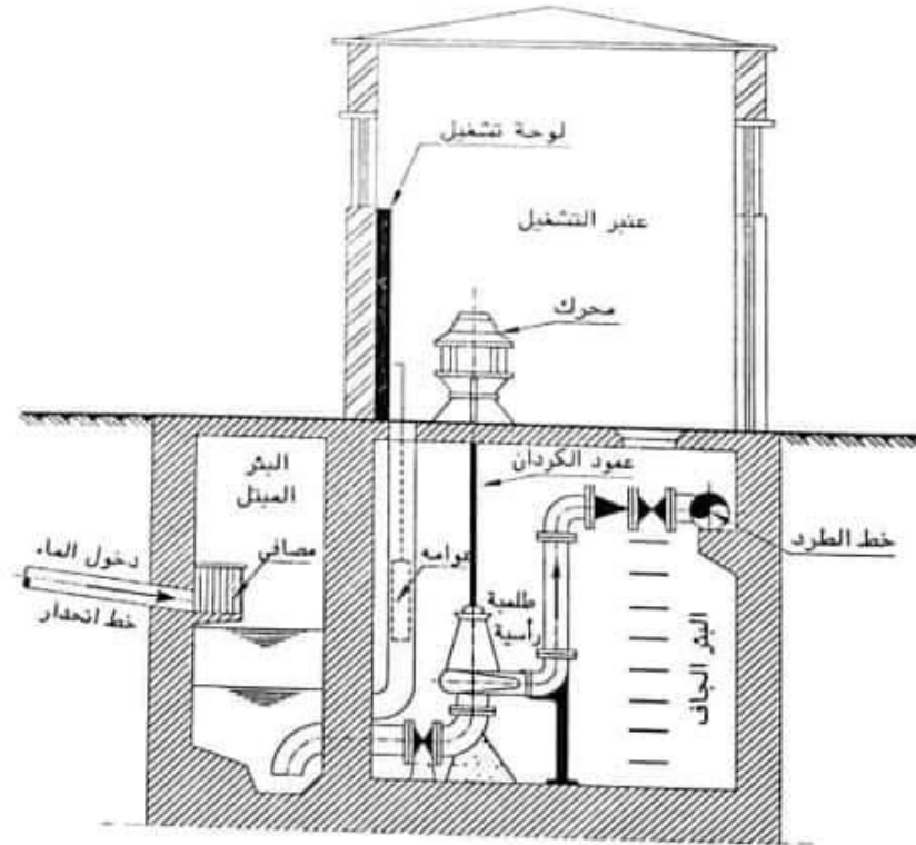
شكل رقم (٤-٣): محطة رفع ذات بئر جاف وآخر مبدل وطمبات رأسية.
