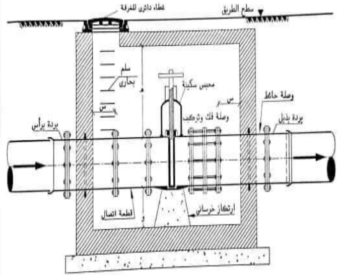
شكل رقم (٧-٣): مقطع رأسي في نموذج لغرفة محابس قفل.
