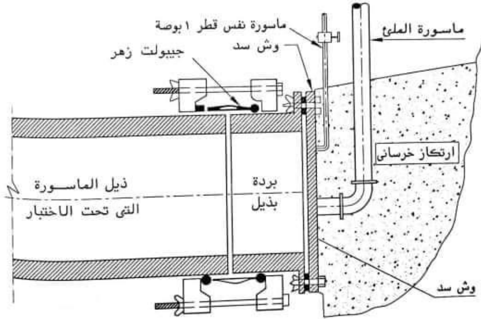
شكل رقم (١٠-٣): تفاصيل النهاية العليا لجزء المواسير المختبر أثناء اختبار بالموقع.
