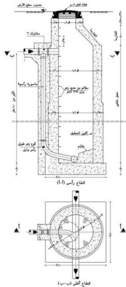
شكل رقم (١٣-٢): مطبق هدار دائري للمواسير ذات القطر حتى ٣٧٥ مم (١٥).
