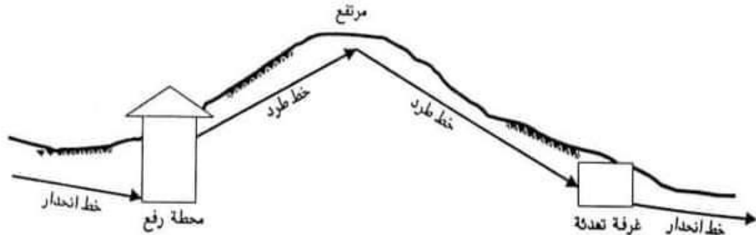
شكل رقم (٣-٢): استخدام محطة رفع وخط طرد وغرفة تهدئة عند اعتراض مرتفع لخط الانحدار.
