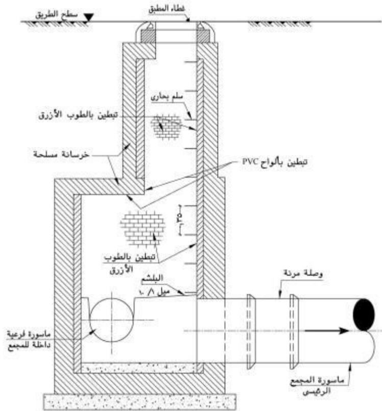
شكل رقم (٩-٢): قطاع رأسي في مطبق من الخرسانة المسلحة المصبوبة في الموقع.
