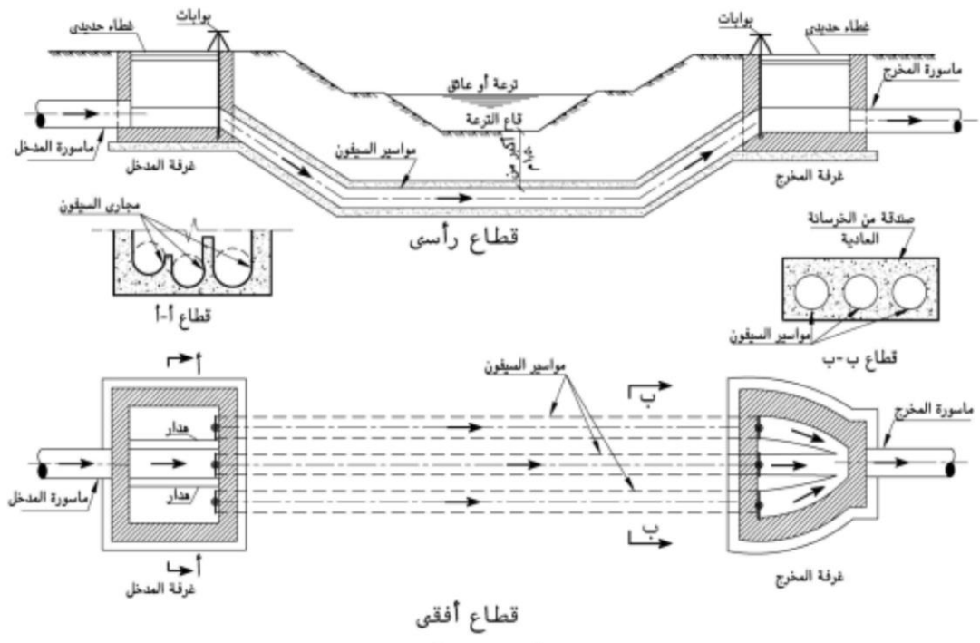
شكل رقم (٢-٢٠): قطاع رأسي ومسقط أفقي في السيفون المقلوب.
