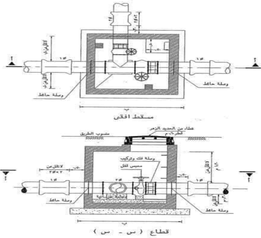
شكل (١-٤) نموذج غرفة محابس قفل
