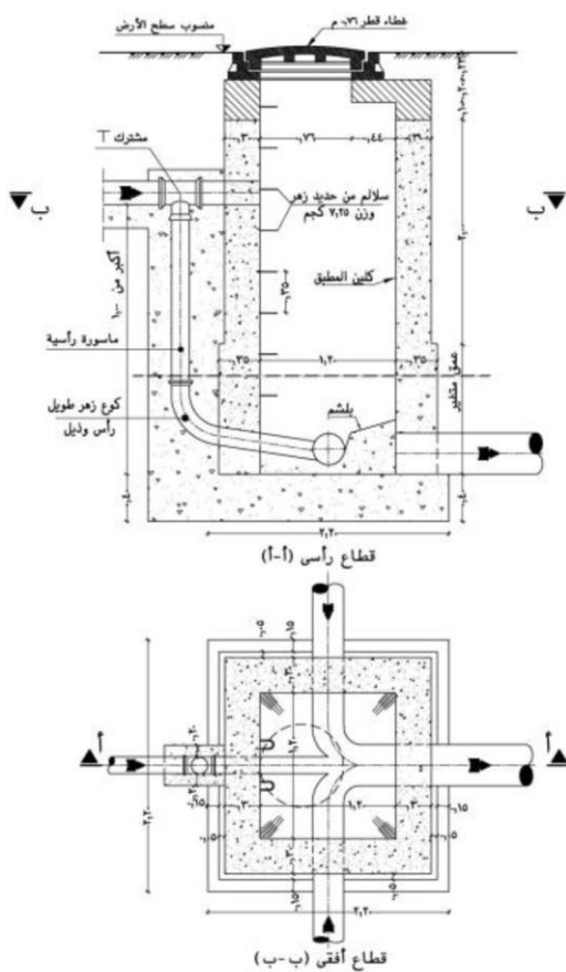
شكل رقم (١٤-٢): مطبق هدار مربع للمواسير ذات القطر أكبر من ٣٧٥ مم (١٥).
