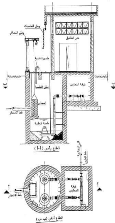
شكل رقم (٥-٣): محطة رفع ذات طلمبات غاطسة.
