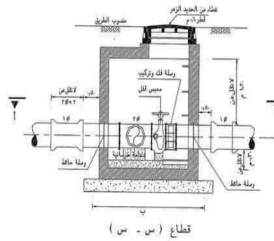
شكل (٤-١) نموذج غرفة محابس قفل
