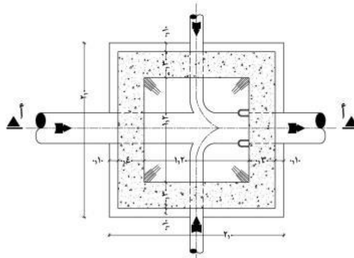
قطاع أفقي (ب-ب)
