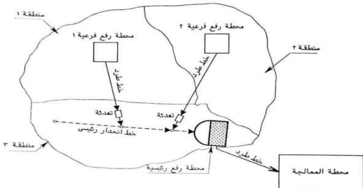
شكل رقم (1-3): تقسيم المدينة إلى مناطق صرف مستقلة واستخدام محطات رفع فرعية ورئيسية.
