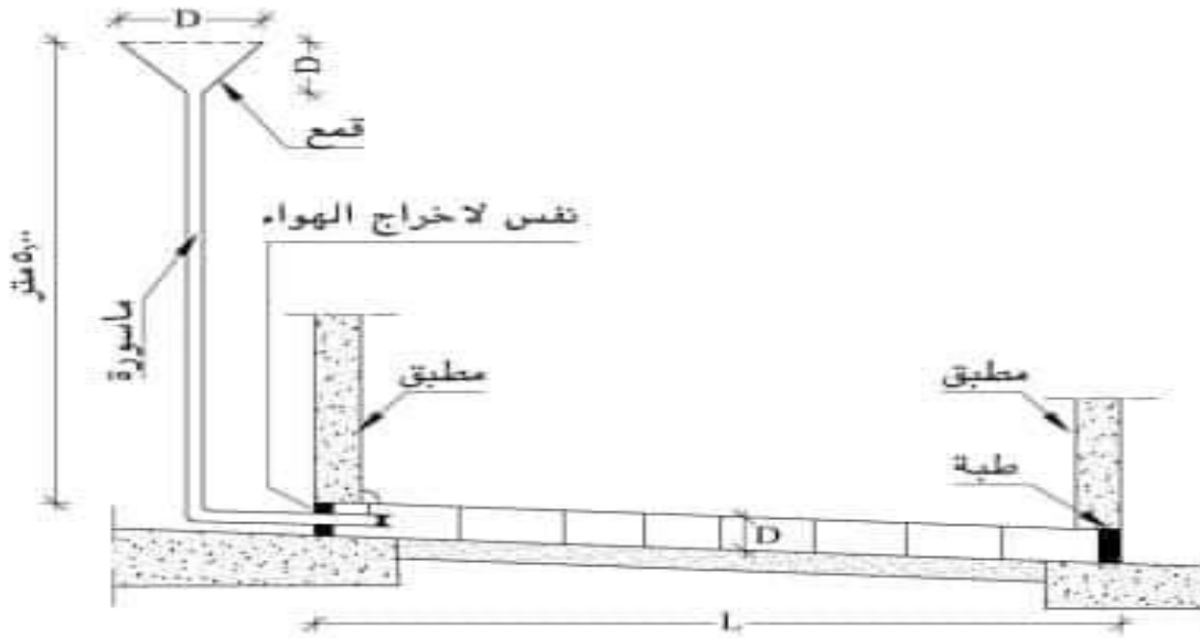
شكل رقم (١-١٦): اختيار القمع لمواسير الصرف الصحي ذات الوصلات المرفقة.
