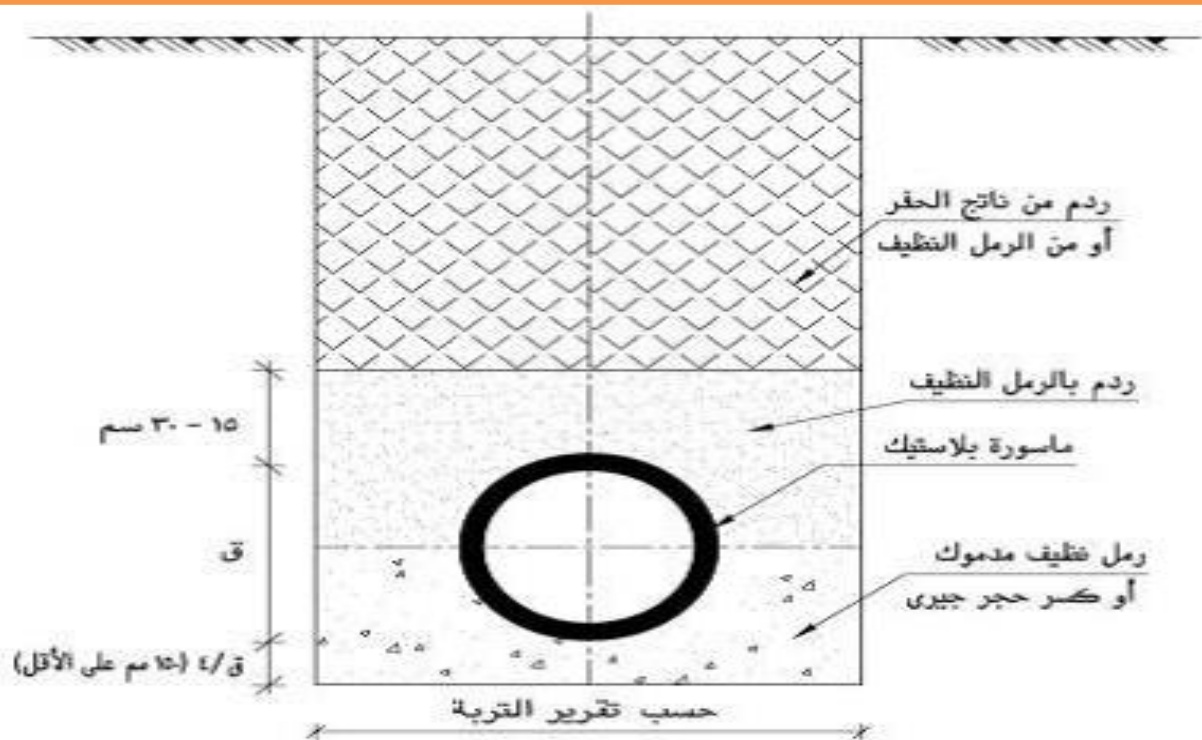
شكل رقم (١٢-١): مثال لقطاع عرضي في أساس مواسير البلاستيك غير اللدن (uPVC) والفيبرجلاس (GRP).
