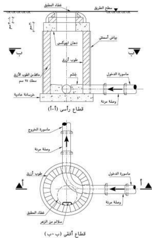
شكل رقم (٢-١٢): تفاصيل مطبق من الطوب الأزرق.
