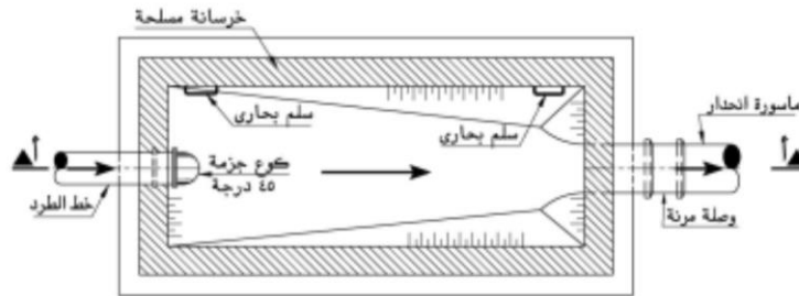
قطاع أفقي (ب-ب)
